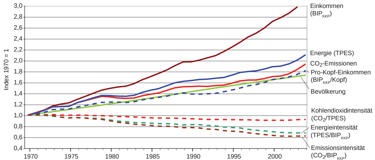
Abbildung SPM.2: relative weltweite Entwicklung von Bruttoinlandsprodukt (BIP) gemessen in KKP (Kaufkraftparität), gesamtener Primärenergieversorgung (TPES), CO 2 -Emissionen (aus der Verbrennung fossiler Brennstoffe, Erdgasabfackelung und Zementherstellung) und Bevölkerung. Zusätzlich zeigt die Abbildung mit gestrichelten Linien pro Kopf-Einkommen (BIP/KKP), Energieintensität (TPES/BIP/KKP), Kohlendioxidintensität der Energieversorgung (CO 2 /TPES) und Emissionsintensität wirtschaftlicher Herstellungsprozesse (CO 2 /BIP/KKP) für den Zeitraum von 1970–2004. [Abbildung 1.5]
