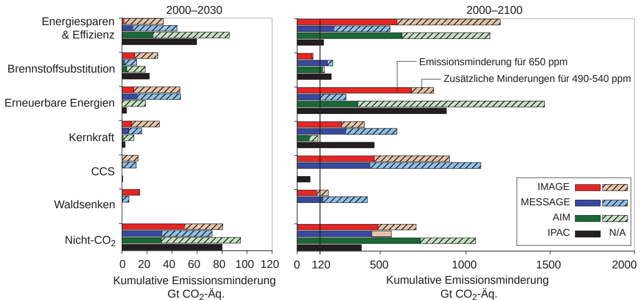
Abbildung SPM 9: Kumulative Emissionsminderungen für unterschiedliche Emissionsminderungsmaßnahmen für 2000 bis 2030 (linke Grafik) und für 2000 bis 2100 (rechte Grafik). Die Abbildung zeigt beispielhafte Szenarien aus vier Modellen (AIM, IMAGE, I-PAC und MESSAGE), die jeweils auf eine Stabilisierung bei 490–540 ppmv CO 2 -Äq. bzw. bei 650 ppmv CO 2 -Äq. abzielen. Dunkle Balken geben die Minderungen für das Ziel von 650 ppmv CO 2 -Äq. an, helle Balken weisen auf die zusätzlichen Reduktionen hin, die notwendig sind, um 490–540 ppmv CO 2 -Äq. zu erreichen. Es ist zu beachten, dass einige Modelle Emissionsminderungen durch die Erweiterung von Waldsenken (AIM und IPAC) oder CCS (AIM) nicht mit einbeziehen, und dass der Anteil an kohlendioxidarmen Energieoptionen an der gesamten Energieversorgung auch durch die Einbeziehung dieser Optionen im Referenzszenario bestimmt wird. CCS schließt Kohlendioxidabtrennung und –speicherung aus Biomasse mit ein. Waldsenken schließen die Minderung von Emissionen aus Entwaldung mit ein. [Abbildung 3.23]
