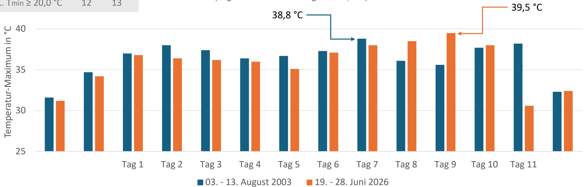
Tageshöchstwerte Temperatur (beginnend mit erstem Tag über 35,0 °C)
