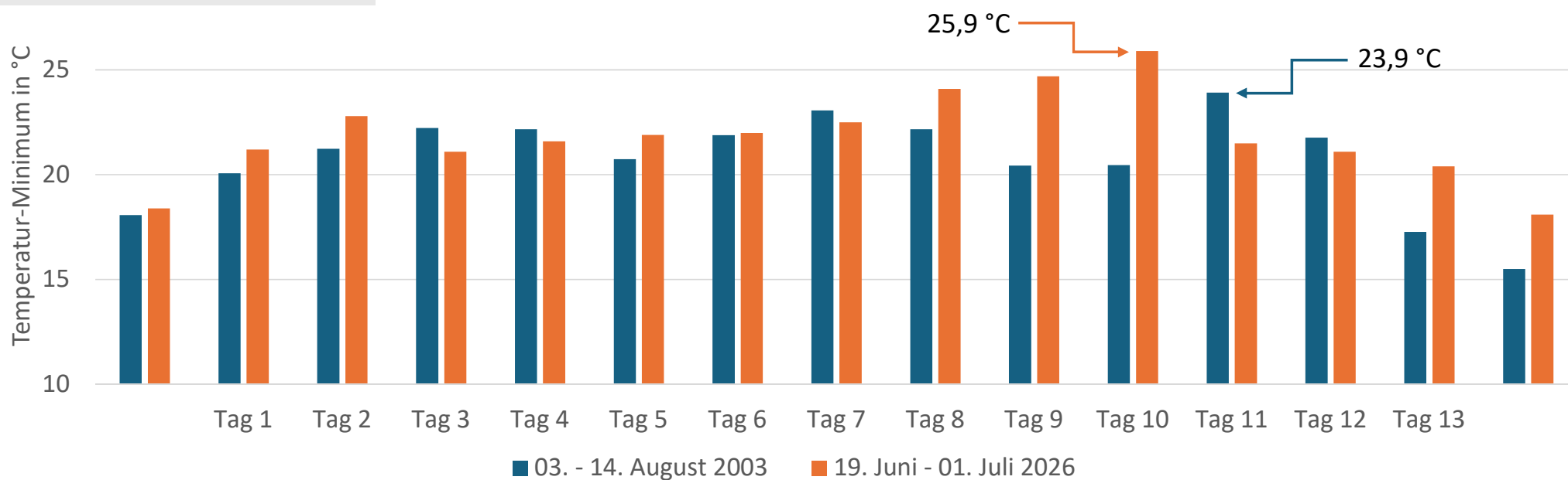
Tagestiefstwerte Temperatur (beginnend mit erstem Tag nicht unter 20,0\text{ °C} )
